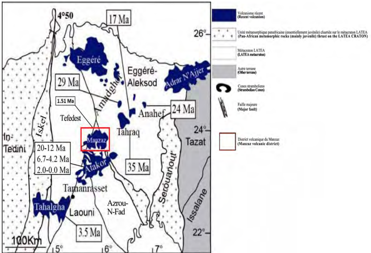
Fig. 2 - Terranes du Hoggar central, principaux districts volcaniques et âges des formations volcaniques (d'après Aït-Hamou et al. , 2000, Benmessaoud, 2014 modifié).
