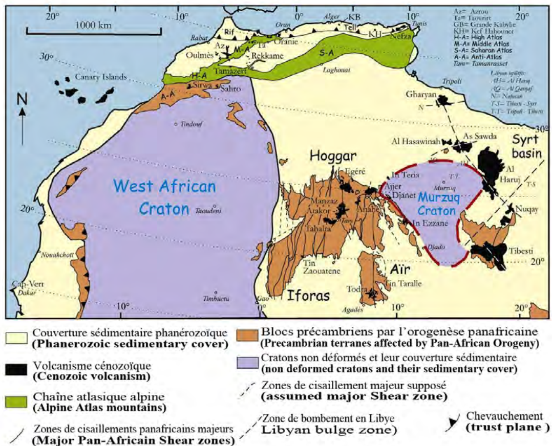
Fig. 1 - Bouclier Touareg et principales provinces volcaniques cénozoïques en Afrique du Nord (d'après Liégeois et al. , 2005).
