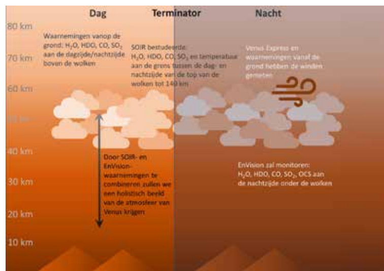
Schema dat de waarneembieden van de verschillende instrumenten weergeeft: SOIR boven de wolken aan de terminator (de grens tussen dag en nacht), telescopen vanaf de aarde boven de wolken zowel overdag als 's nachts en EnVision onder de wolken, eveneens de hele dag en nacht door. Daarnaast worden ook de gassen vermeld die door deze instrumenten worden gemonitord.
