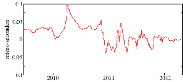
Figuur 3. Gedrag van UTC(ORB) ten opzichte van UTC over de laatste drie jaar.
