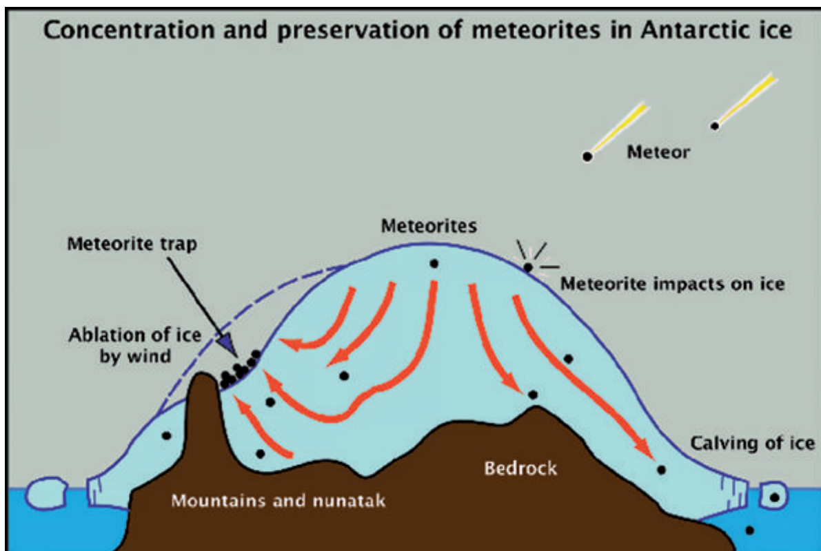
Schéma 1: Accumulation, progression et préservation de la météorite dans les champs de glace bleue.
