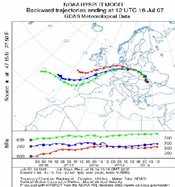
Fig. 9 - HYSPLIT back trajectories
