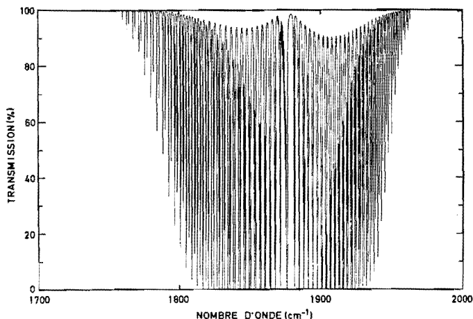
FIG. 2. — Spectre d'absorption à résolution infinie du monoxyde d'azote entre 1700 et 2000 \text{cm}^{-1} calculé pour une cellule de 1 cm de long contenant NO à la pression de 1 atmosphère et à la température de 300 °K.
