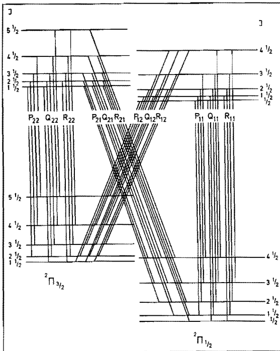
FIG. 1. — Schéma général montrant toutes les transitions possibles entre les niveaux de deux états {}^2\Pi(a) . Les échelles ne sont pas respectées. Le dédoublement lambda, très faible, n'est pas représenté, afin de ne pas surcharger la figure.
