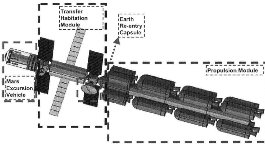
Fig.2 : Représentation du train spatial au départ de la Terre, la longueur totale en est de 102 m. La capsule de rentrée est le seul module pour lequel le rapport ne donne pas d'étude détaillée. (Rapport ESA)
