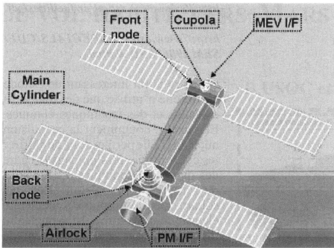
Fig.4 : Le module de transfert et d'habitation. MEV signifie Mars Exploration Vehicle et PM : Propulsion Module. Ce module se compare à un assemblage d'éléments de la station spatiale internationale. Il reprend notamment le concept de la coupole d'observation et de navigation, nécessaire à la fois du point de vue technique et psychologique. (Rapport ESA)
